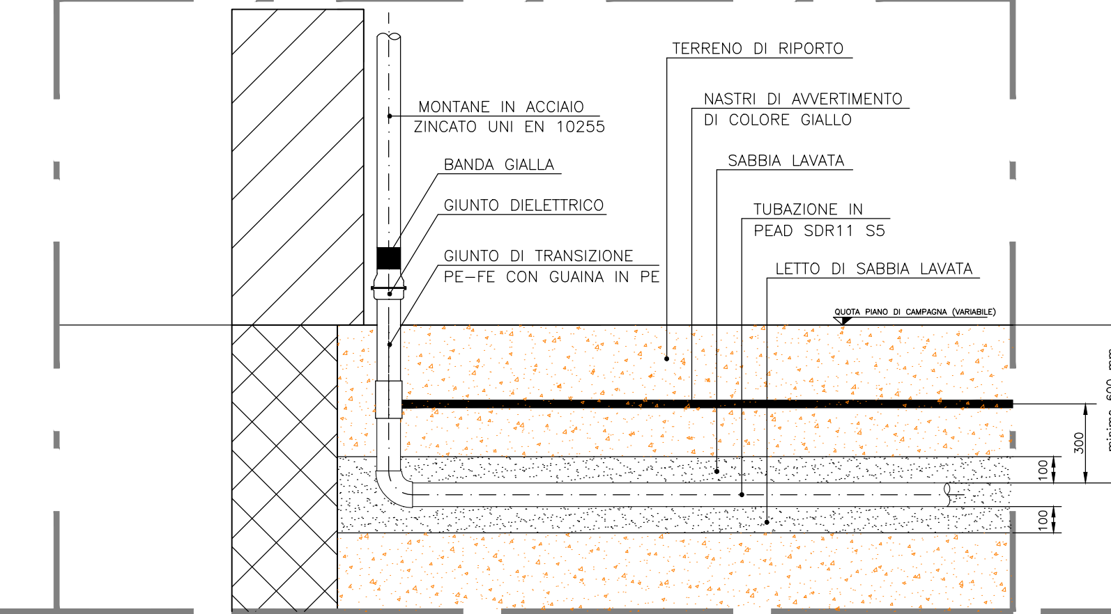
PARTICOLARE COLLEGAMENTO TUBAZIONI DA POLIETILENE IN ACCIAIO ZINCATO
